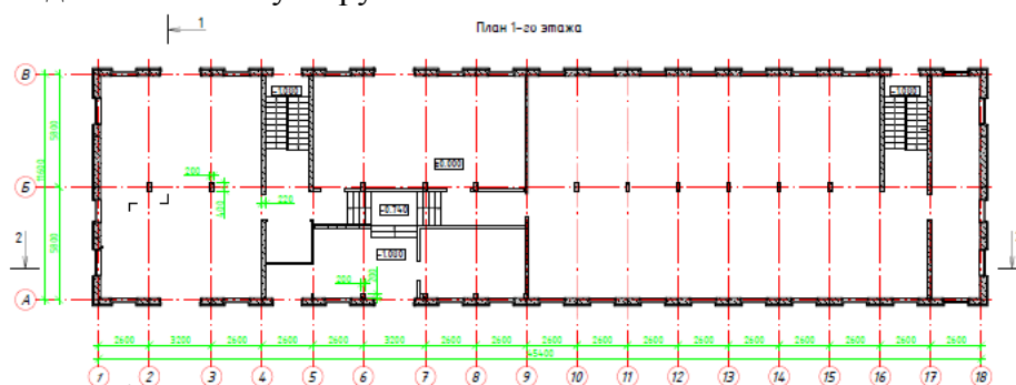
Рис.2. План здания
