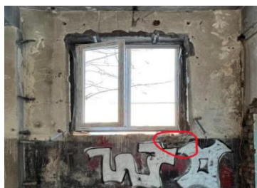
Рис. 6. Трещины по внутреннему слою штукатурного покрытия: а - стеновая панель в осях 9-10/В на отм. +2,700 (2 этаж); б - стеновая панель в осях 8-9/В на отм. +5,400 (3 этаж)
