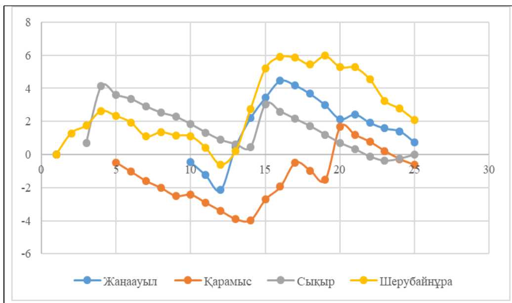
Сурет 1 Нұра өзені салаларының 1970 жылдарға дейінгі айырымдық интеграл қисығы
