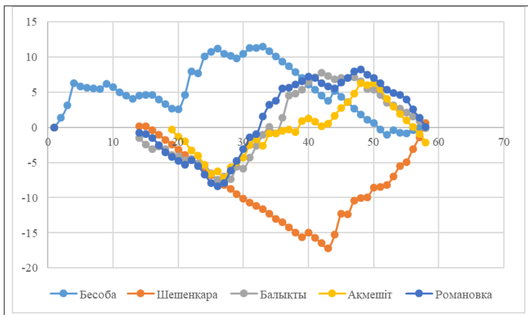
Сурет 2 Нұра өзені бойындағы бекеттердің 1970 жылдардан кейінгі айырымдық интеграл қисығы
