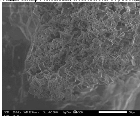
Сурет 2. Синтезделген MgO үлгісінің SEM суреттері.
