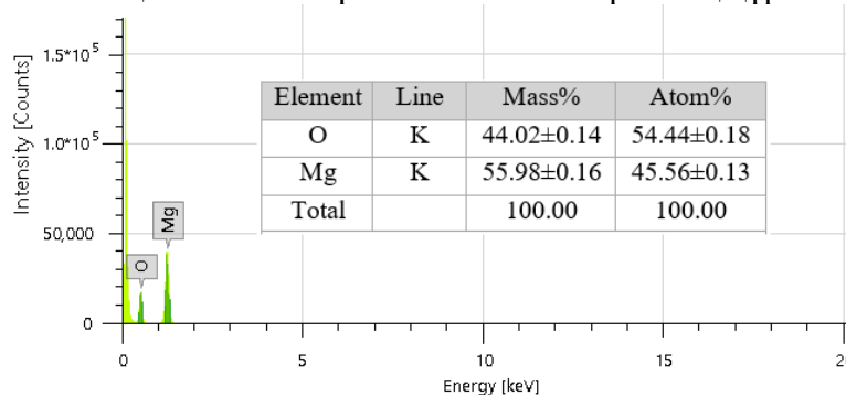
Сурет 3. MgO үлгісінің элементтік талдауы.
