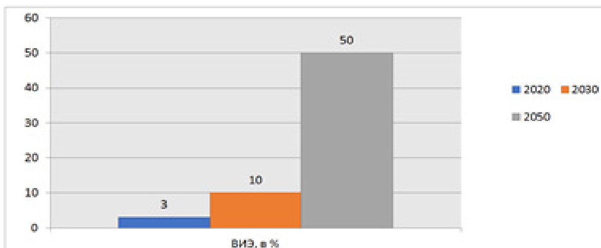
Рисунок 2. Прогноз развития в Казахстане ВИЭ и выработке электроэнергии на этих источниках 1
